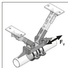
Punkt stały typ A z uchwytami przegubowymi (montaż)
